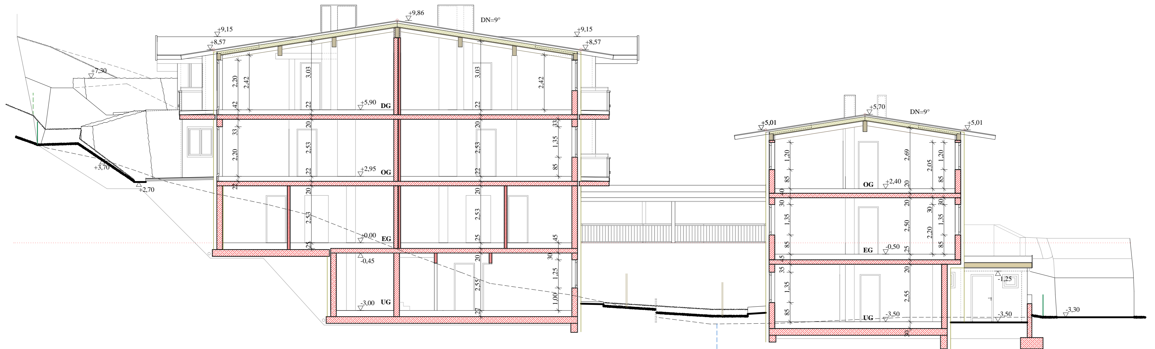
SCHNITT B - B
